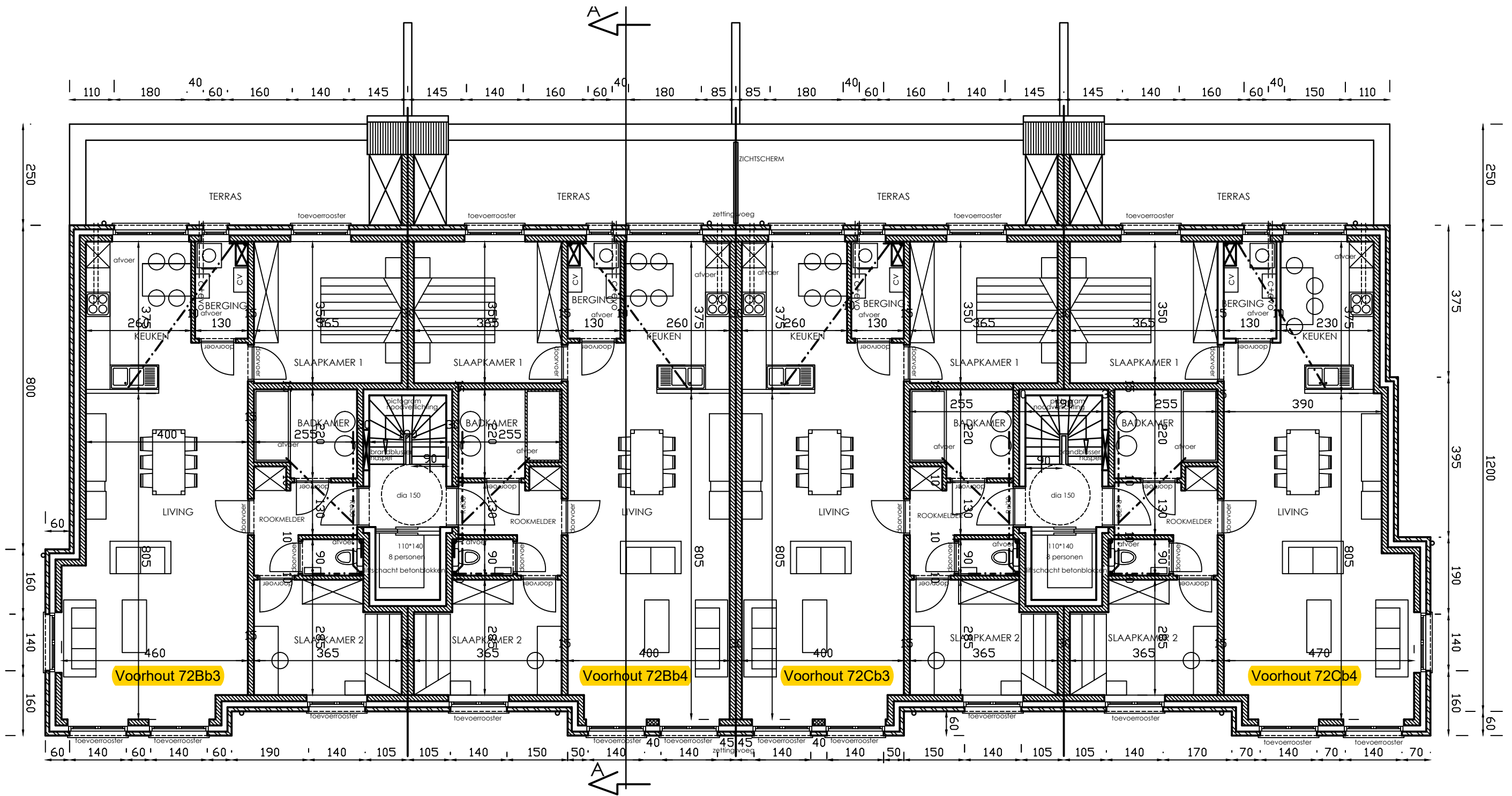
EERSTE VERDIEPING
